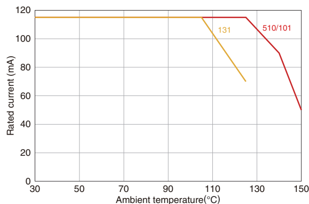
额定电流温度特性 (额定值降低)
